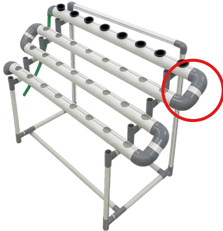
NFT (Nutrient Film Technique)
