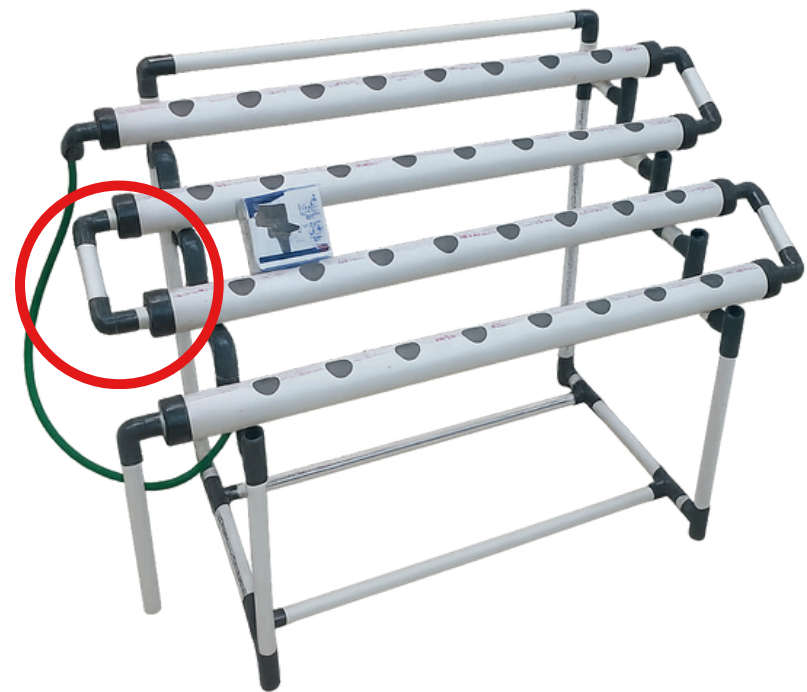
DFT (Deep Flow Technique)
